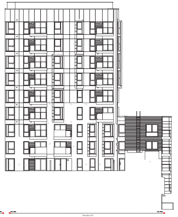
Elevation E4
